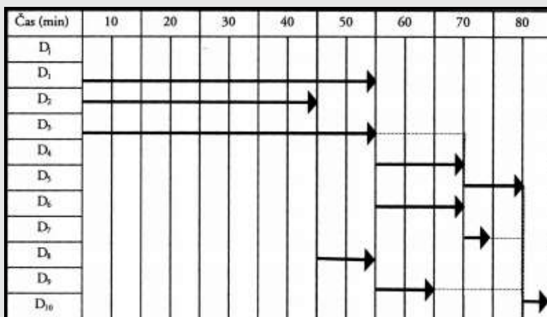
Diagram 4.1: Časovni mrežni diagram za odpremo potniškega letala.
